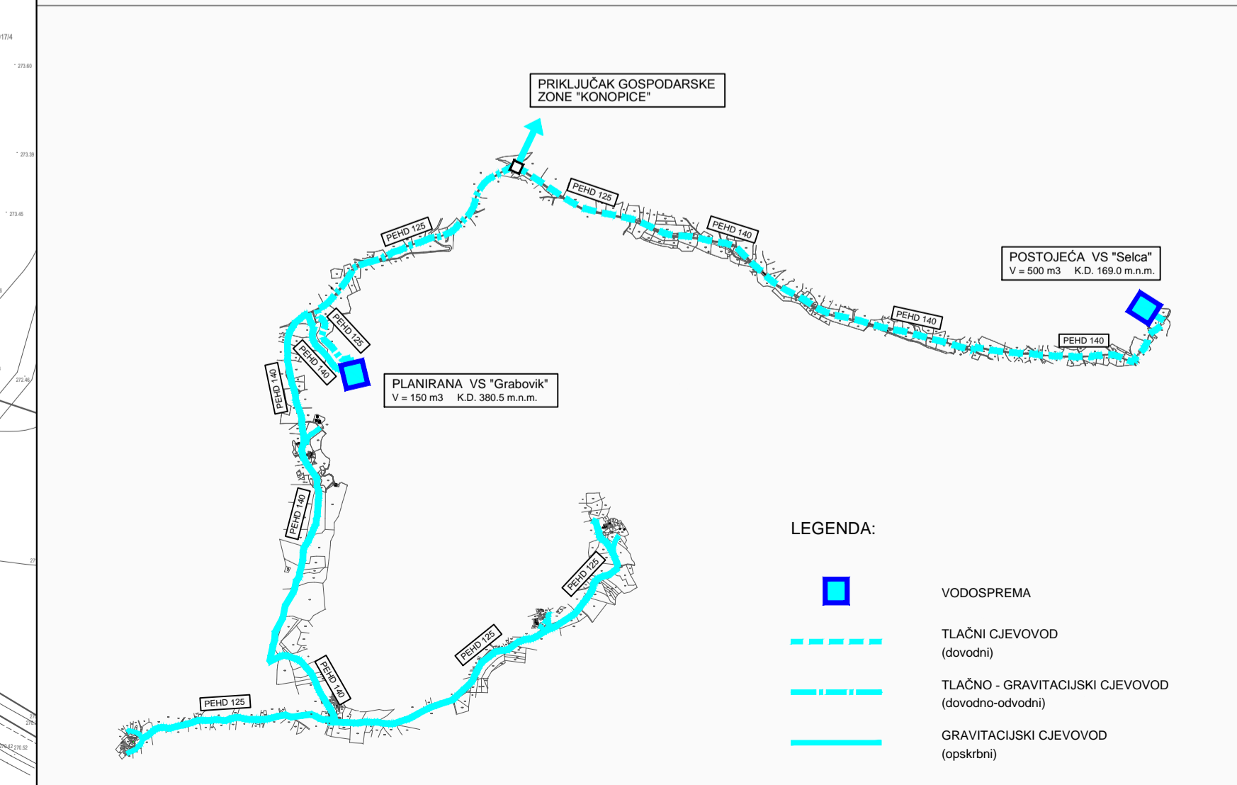
SHEMA VODOOPSKRBE šireg područja gospodarsko poslovne zone "Konopice"
